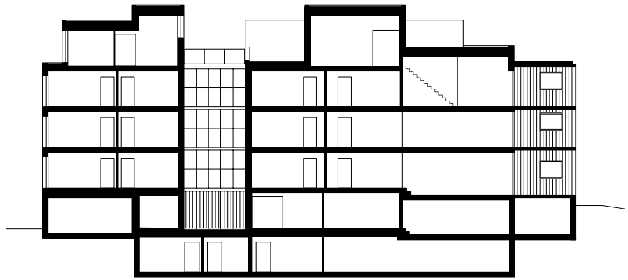
Längsschnitt
