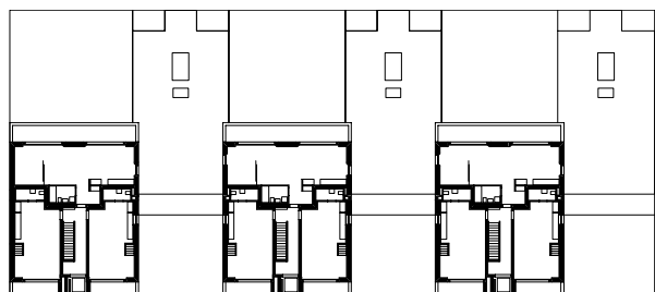
5. Obergeschoss
